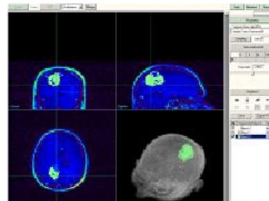
Fig. 3. UbiCAS Server.
